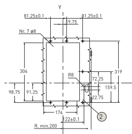
3 Размеры с отметки и сверления
